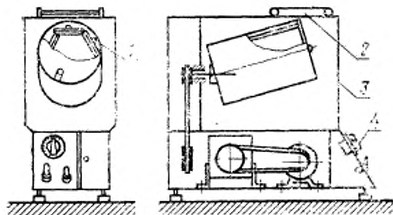
1—пластины; 2—воронштейн для заправки элементарных проб; 3—вращающаяся камера; 4—часовое реле
