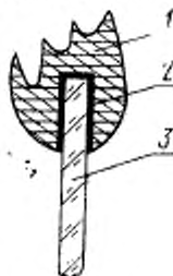
1—резиновый уплотнитель; 2—мастика; 3—стекло
