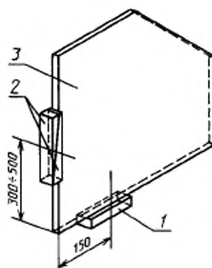
1 — опорная подкладка; 2 — фиксирующая подкладка; 3 — светопрозрачное заполнение; 4 — нестепрозрачное заполнение
