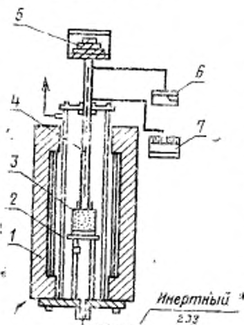
1—нагревательная печь; 2—нагревательная камера; 3—тигель с пробой; 4—шток с подпятником; 5—груз; 6—устройство регулирования и контроля температуры нагрева пробы; 7—прибор для автоматической записи температуры пробы и перемещения штока
