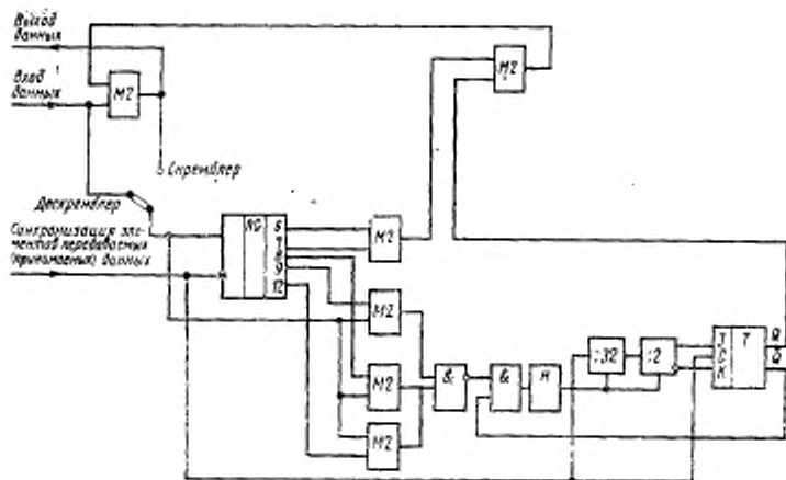
Функциональная схема скремблера-дескремблера для УПС-4,8 ТЧ
