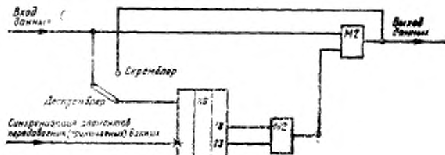
Функциональная схема скремблера-дескремблера для УПС-9,6 ТЧ
