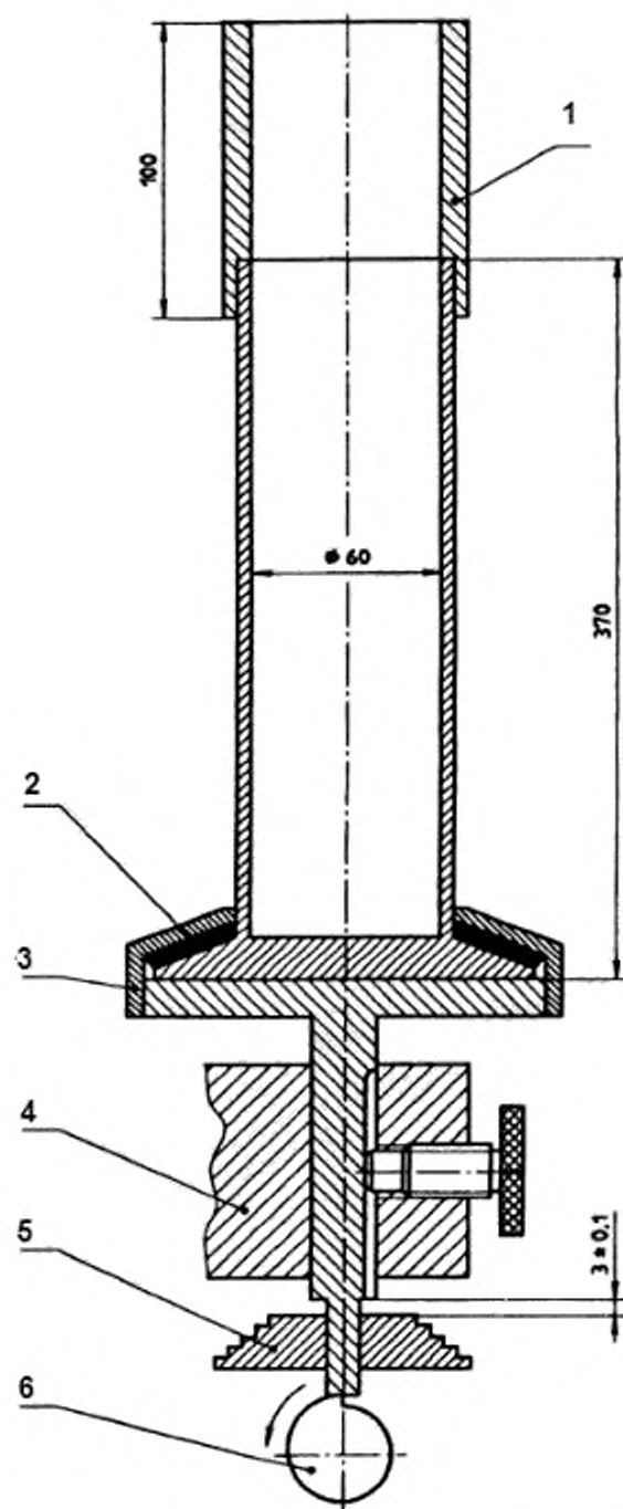
1 – кольцо; 2 – резиновое уплотнение; 3 – держатель измерительного цилиндра с направляющим зажимом; 4 – штангенциркуль; 5 – опора; 6 – кулачковый вал
