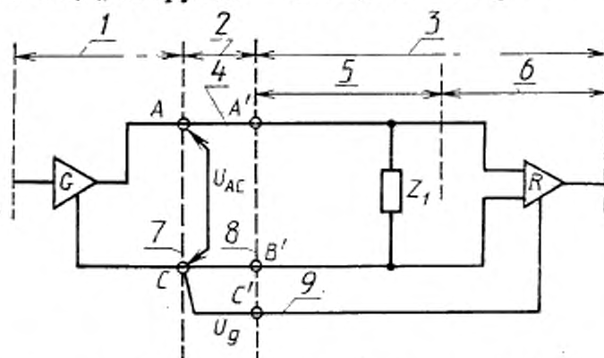
1—генератор; 2—соединительный кабель; 3—нагрузка; 4—сигнальный провод; 5—схема согласования; 6—приемник; 7—точка стыка генератора; 8—точка стыка нагрузки; 9—сигнальное заземление; U_{AC} —выходное напряжение генератора; U_g —разность потенциалов заземления; A—активная точка стыка генератора; C—точка сигнального заземления генератора; A'—активная точка стыка нагрузки; B'—точка сигнального заземления нагрузки; C'—нулевая точка приемника; Z_1 —согласующее сопротивление (применяемое только для окончания коаксиального кабеля).
