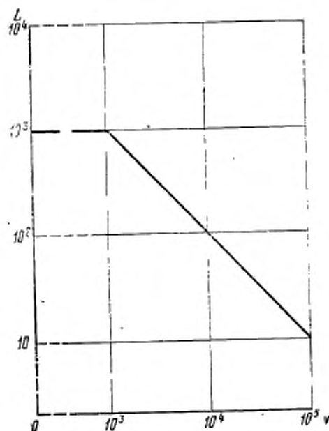
Зависимость длины кабеля от скорости передачи для несимметричной цепи стыка
