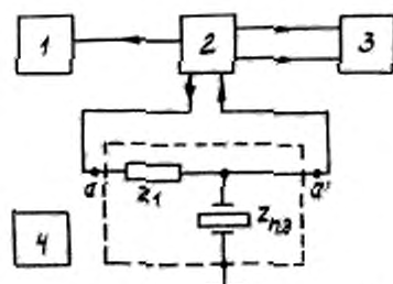
1 — частотометр; 2 — измеритель АЧХ; 3 — графопостроитель; Z_{н.з} — проверяе- мый ПЭП; Z_1 — электрическая нагруз- ка; 4 — акустическая нагрузка
