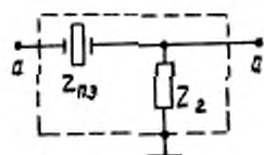
Z_{н.з} — проверяемый ПЭП; Z_2 — электрическая нагруз- ка
