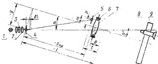
1 — источник света, 2 — конденсор; 3 — светофильтр; 4 — раздвижная щель; 5 — диафрагма с парой параллельных щелей; 6 — объективодержатель; 7 — испытуемый объект; 8 — микроскоп; 9 — поперечная линейка
