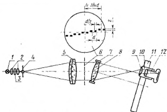
1 — источник света; 2 — конденсор; 3 — светофильтр; 4 — раздвижная щель; 5 — объектив коллиматора; 6 — многощелевая диафрагма; 7 — объективодержатель; 8 — испытуемый объект; 9 — цилиндрический окуляр; 10 — каретка; 11 — поперечная линейка; 12 — фотоплават.
