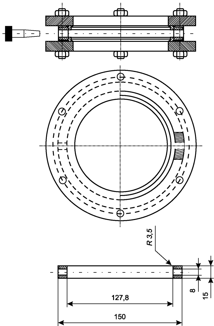
Рисунок С.7 – Камера, тип Е
