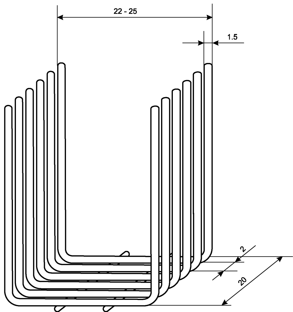
Рисунок С.2 – Штатив для образцов
