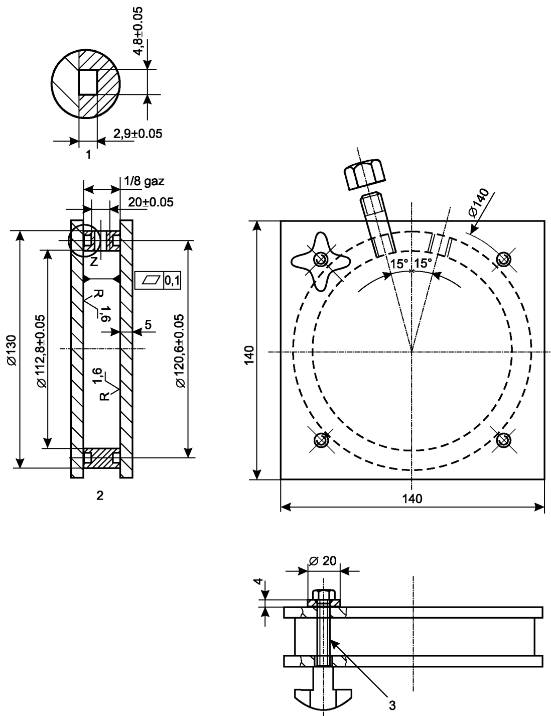
1 – деталь Z; 2 – уплотнительное кольцо \varnothing 117,07 / 124,13 / 3,53 ; 3 – винт НМF-50
