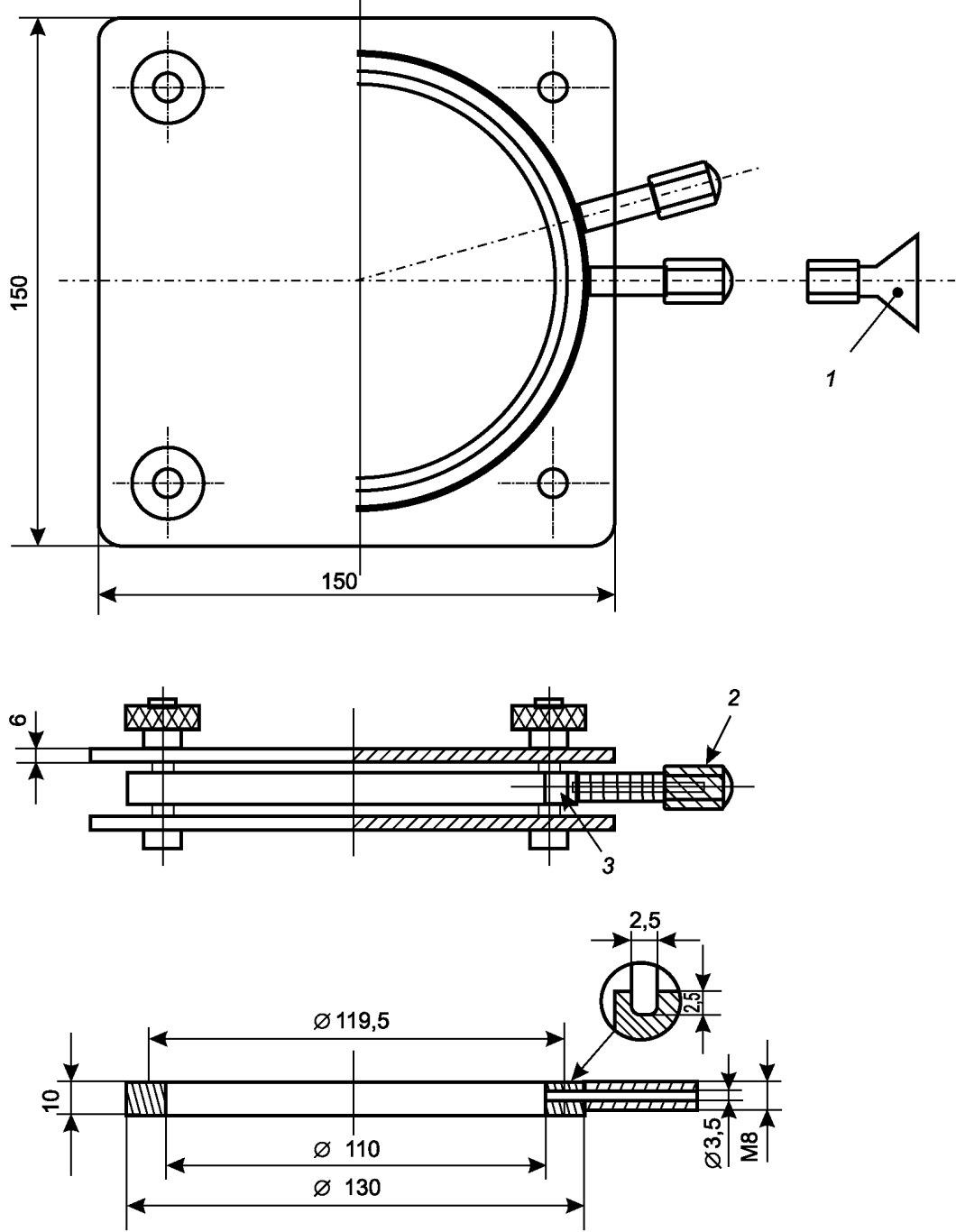
1 – воронка для заполнения; 2 – диск из ПТФЭ; 3 – уплотнительное кольцо из ПТФЭ (119,5 × \varnothing 3 ) Рисунок С.4 – Камера, тип В
