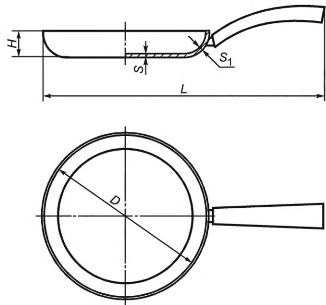
Рисунок 2 — Круглая сковорода с одной ручкой
