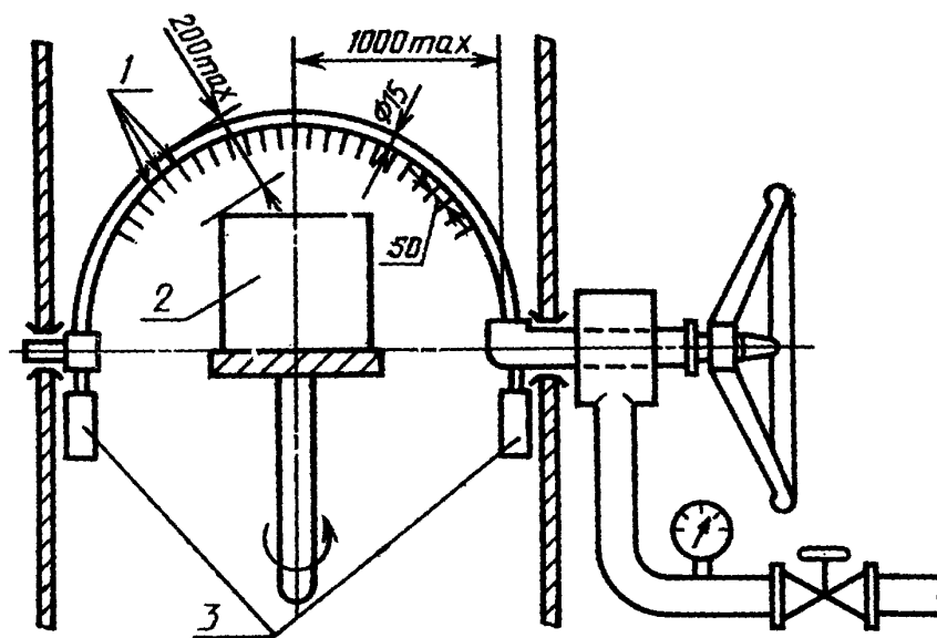
1 — отверстия диаметром 0,4 мм; 2 — испытуемое оборудование; 3 — противовесы.
