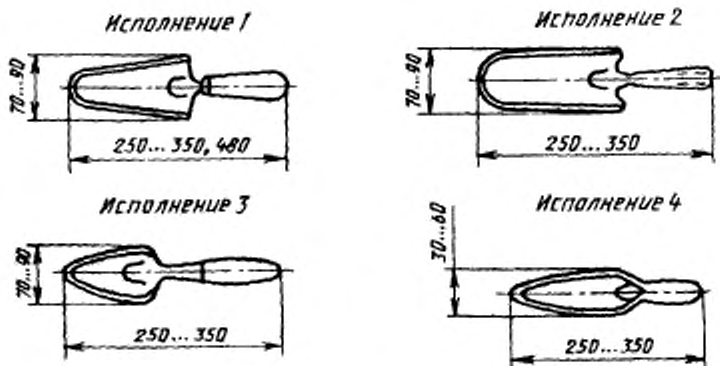
Рисунок 1 — Посадочный совок
