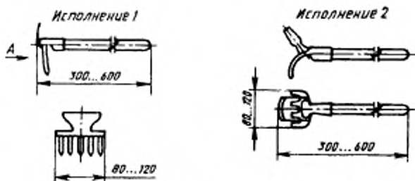
Рисунок 6 — Комбинированный рыхлитель
