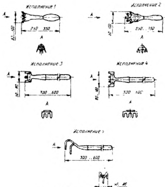
Рисунок 5 — Рычаг, лист 1
