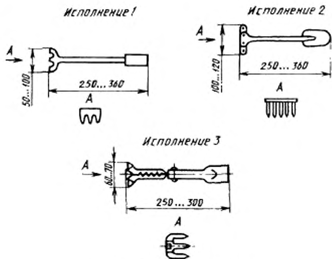
Рисунок 3 — Грабли-лопатка
