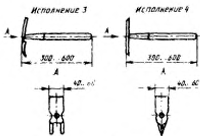
Рисунок 4. лист 2
