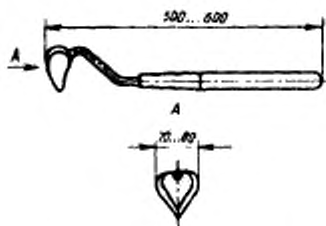
Рисунок 8 — Бороздовичок
