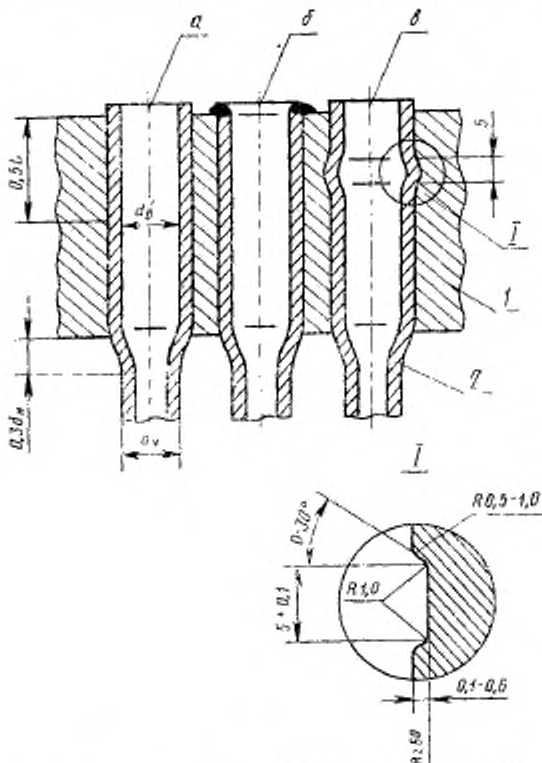
Конструкция соединений труб с трубными решетками
