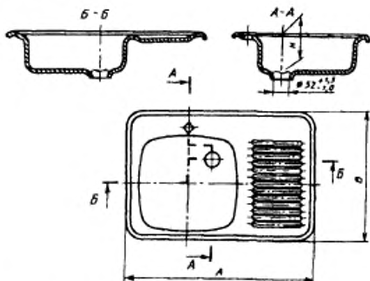
Рисунок 9 — Мойка стальная эмалированная с одной чашей со сливной полкой встраиваемая (тип МСВП)
