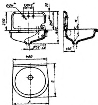
Рисунок 11 — Раковина стальная эмалированная (типы РСУ-1 и РСУ-2)
