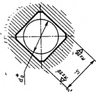
* Диаметр отверстия до протягивания (для справок).
