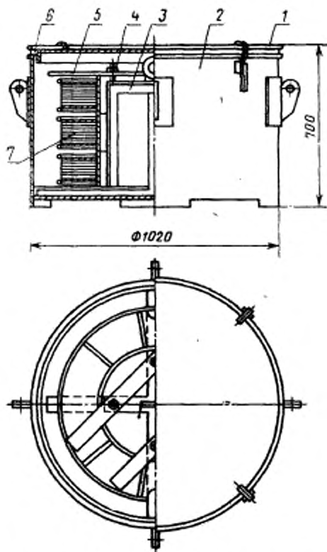
1—крышка; 2—корпус; 3—поддон; 4—гайка; 5—шайба; 6—прокладка; 7—порошковая лента в кассете
