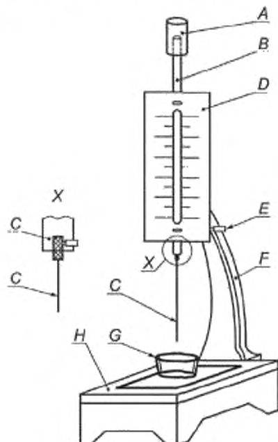
A — дополнительная нагрузка; B — стержень; C — игла Вика; D — градуированная шкала; E — винтовой зажим; F — поддерживающая опора; G — конусная цилиндрическая форма; H — основание пластины
