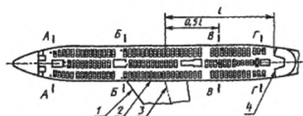
А, В, Г — сечения; 1 — передняя кромка крыла; 2 — корневая нервюра; 3 — задний лонжерон; 4 — задняя стенка пассажирской кабины
