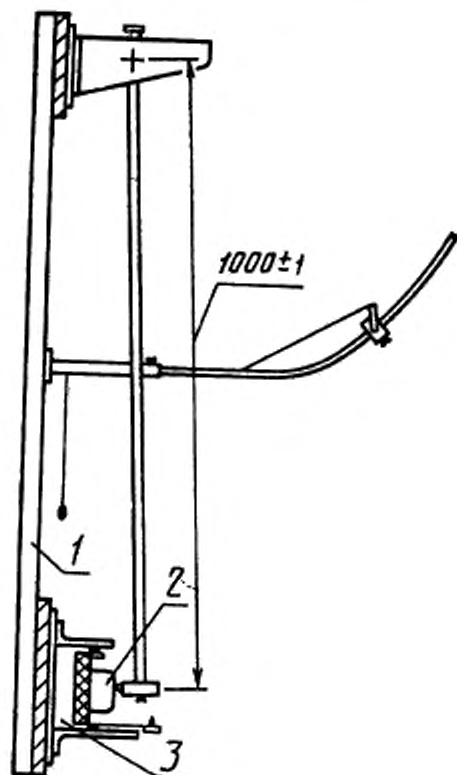
1—каркас; 2—образец; 3—монтажная опора
