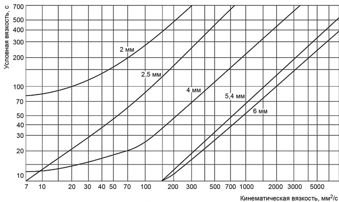
Рисунок Б.1 — Зависимость условной вязкости материала ( \varsigma ) от кинематической вязкости ( \text{мм}^2/\text{с} ) в вискозиметрах с различным диаметром сопла
