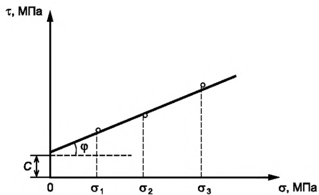
а) График \tau=f(\sigma)
