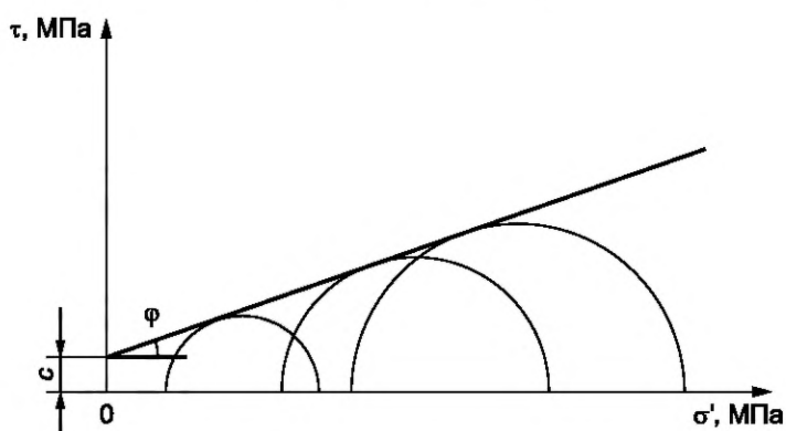
Рисунок Ж.1.2 — Диаграмма прочности Кулона — Мора
