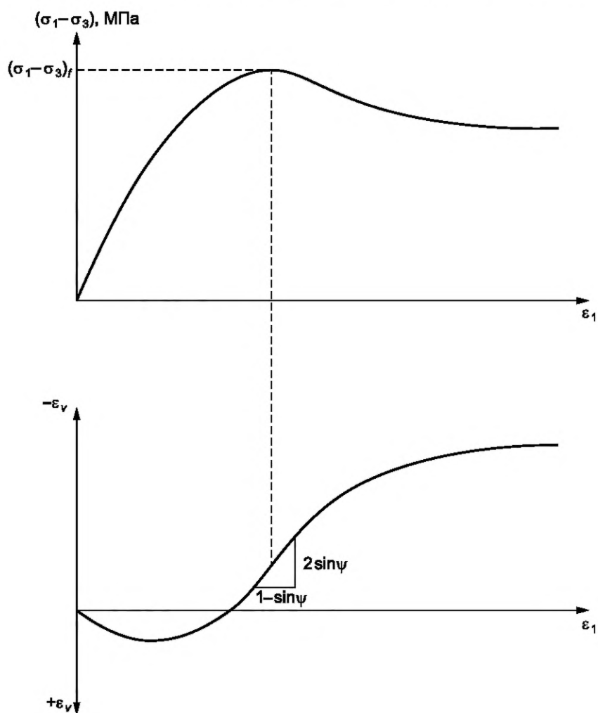
Рисунок К.1 — График к определению угла дилатансии
