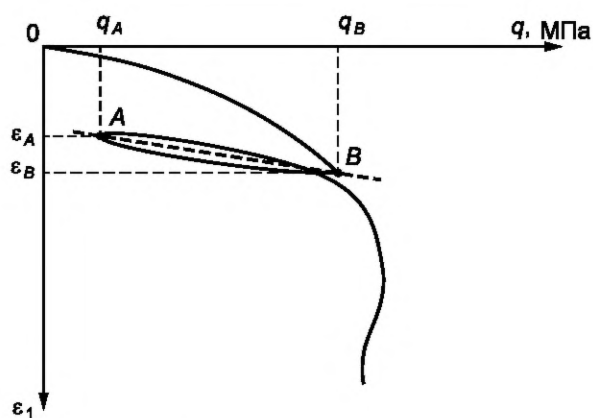
Рисунок Ж.2.3 — Иллюстрация графического определения модуля повторного нагружения E_{ur}
