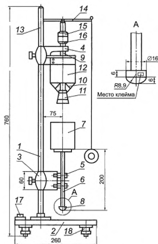
1 — штатив; 2 — основание; 3 — подвижный кронштейн; 4 — неподвижный кронштейн; 5 — ролики; 6 — шток с площадкой; 7 — стакан для приемки груза; 8 — грибовидная насадка; 9 — направляющая; 10 — запорный шток; 11 — пробка; 12 — грузовой стакан с отверстием в коническом дне; 13 — ось; 14 — рычаг; 15 — колпачок; 16 — гайка; 17 — уровень; 18 — регулировочные ножки
