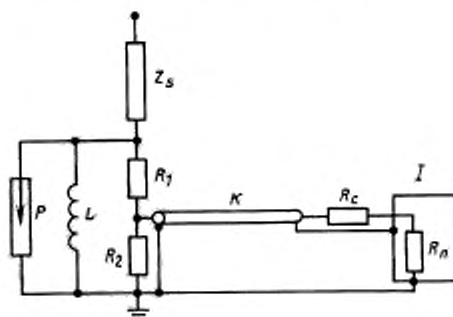
I — измерительный прибор с входным сопротивлением R_n ; K — радиочастотный кабель; P — разрядник; Z_s — элемент связи; L — катушка индуктивности; R_c — резистор, согласующий вход измерительного прибора с волновым сопротивлением кабеля; R_1 и R_2 — резисторы
