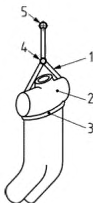
1 – спасательная петля; 2 – манекен корпуса человека; 3 – основная лямка; 4 – элемент подвеса; 5 – элемент крепления
