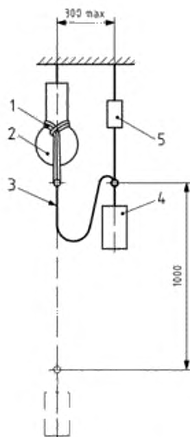
1 – спасательная петля, 2 – тест-форма, 3 – испытательная стропа, 4 – испытательная масса, 5 – устройство быстрого расцепления
