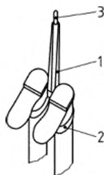
1 – спасательная петля, 2 – основная лямка, 3 – элемент крепления
