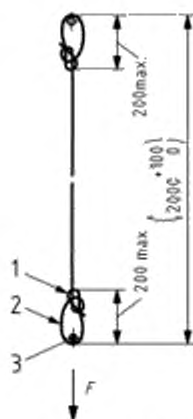
Рисунок 6 – Испытательная стропа для проверки прочности динамической нагрузкой
