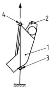
1 – спасательная петля; 2 – манекен корпуса; 3 – нижнее кольцо манекена корпуса; 4 – элемент крепления
