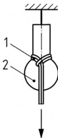
1 – спасательная петля; 2 – испытательная форма
