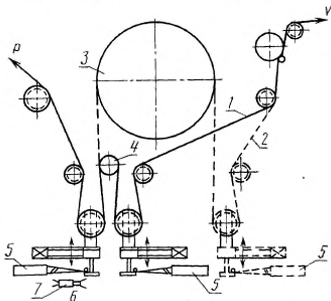
Аппаратура для определения коэффициента динамического трения
