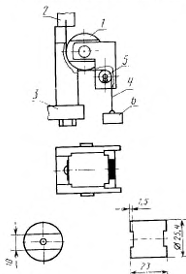
1—контртело; 2—измерительный зажим динамометрического прибора; 3—подвижной зажим; 4—магнитная левка; 5—направляющий ролик; 6—груз (65 г)
