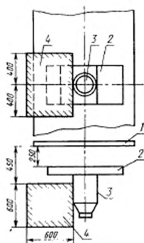
1—опорная стенка поворотного стола-штатива; 2—экранно-снимочное устройство или экранодержатель, либо панель крепления УРИ; 3—усилитель рентгеновского изображения (УРИ); 4—зона защиты
