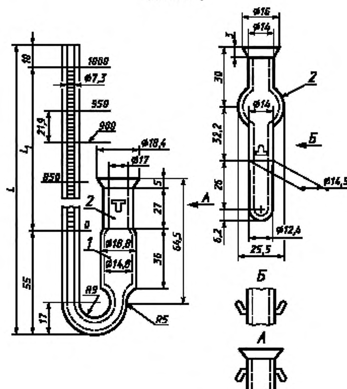
1 — корпус с градуированной трубкой; 2 — пробка
