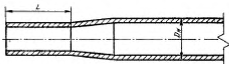
Калиброванный конец трубы
