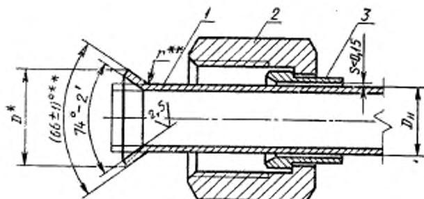
Калиброванный конец трубы
