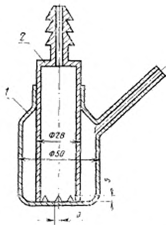
1—полиэтиленовая банка БИЛ-100; 2—цилиндр из фторопласта
