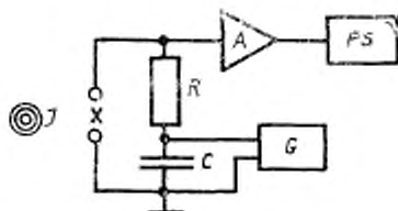
I —источник ионизирующего излучения; X —входные выводы устройства; R —резистор утечки; C —блокирующий конденсатор; A —усилитель; G —источник рабочего напряжения; PS —измеритель временных интервалов
