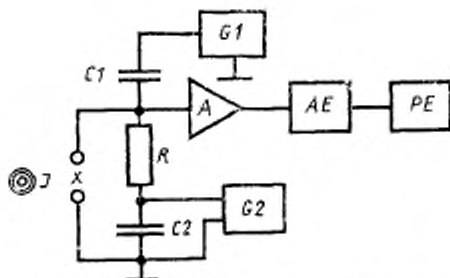
I —источник ионизирующего излучения; X —выходные выводы установки; C1 —дозиметрический конденсатор; R —резистор утечки; C2 —блокирующий конденсатор; G1 —генератор импульсов напряжения; A —ЗУ; G2 —источник рабочего напряжения; AE —масштабный преобразователь; PE —амплитудный анализатор
