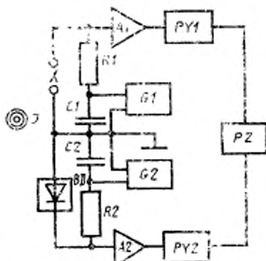
1—источник импульсов понизирующего излучения; X—входные выводы установки; BD—ППД-монитор; R1, R2—резисторы утечки; G1, G2—блокирующие конденсаторы; A1, A2—зарядочувствительные усилители; G1, G2—источники рабочего напряжения; PY1, PY2—интегрирующие измерители; PZ—измеритель отношений сигналов
