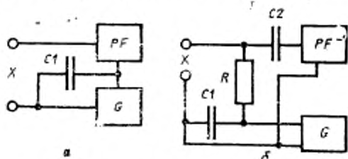
X—входные выводы установки; C1—блокирующий конденсатор; PF—измеритель емкости; G—источник рабочего напряжения; R—резистор утечки; C2—разделительный конденсатор
