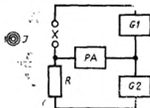
I —источник ионизирующего излучения; X —входные выводы установки; R —компенсационный резистор; PA —измеритель тока; G1 —источник рабочего напряжения; G2 —источник компенсирующего напряжения
