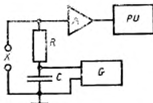
X —выводы для подключения ИПД; R —резистор утечки; C —блокирующий конденсатор; A —ЗУ; G —источник рабочего напряжения; PU —измеритель среднего квадратического значения переменного напряжения
