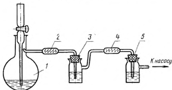
1—реакционная колба; 2, 4—трубки с сжигателем, пропитанным концентрированной серной кислотой; 3—приемник фтора, содержащий 15 см 3 дистиллированной воды; 5—приемник углекислого газа, содержащий 15 см 3 аммиачного раствора хлорида бария
