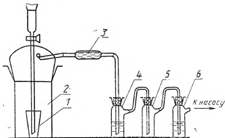
1 — никелевый тигель с охлажденным расплавом, 2 — реакционный сосуд; 3 — трубка с силикагелем, пропитанным концентрированной серной кислотой; 4 — приемник фтора, содержащий 15 см³ дистиллированной воды; 5 — промежуточная емкость; 6 — приемник углекислого газа, содержащий 15 см³ аммиачного раствора хлорида бария
