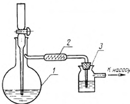
1—реакционная колба; 2—трубка с силикагелем, пропитанным концентрированной серной кислотой; 3—приемник фтора, содержащий 15 см 3 дистиллированной воды
