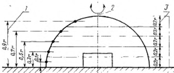
Круговые траектории перемещения микрофонов в горизонтальной плоскости полусферической поверхности
