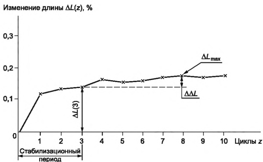
Рисунок 2 — Пример определения формоустойчивости образца
