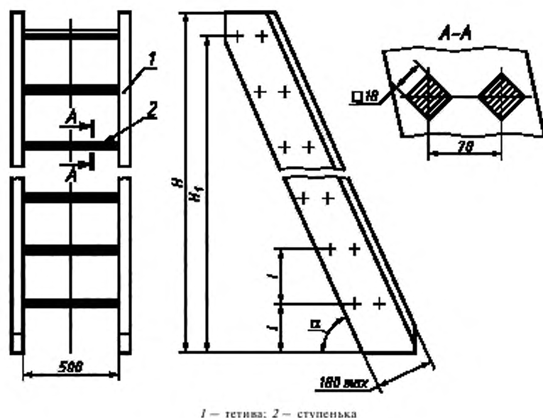
Рисунок 3 — Тип 1, исполнение 1-дп
