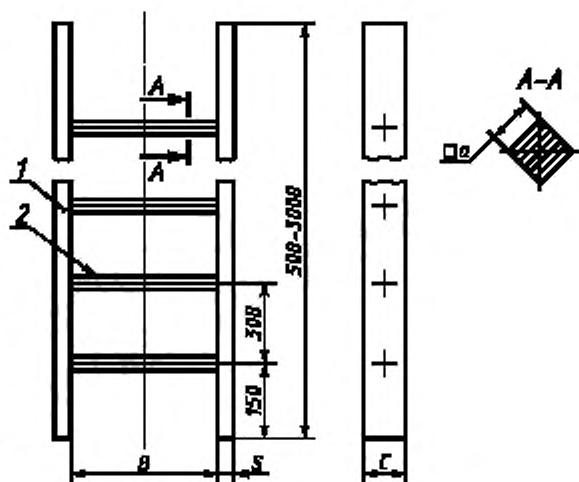
Рисунок 5 — Тип 2, исполнения 2-п, 2-2п
