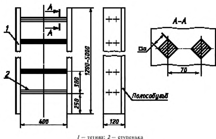
Рисунок 6 — Тип 2, исполнения 2-дп, 2-2дп
