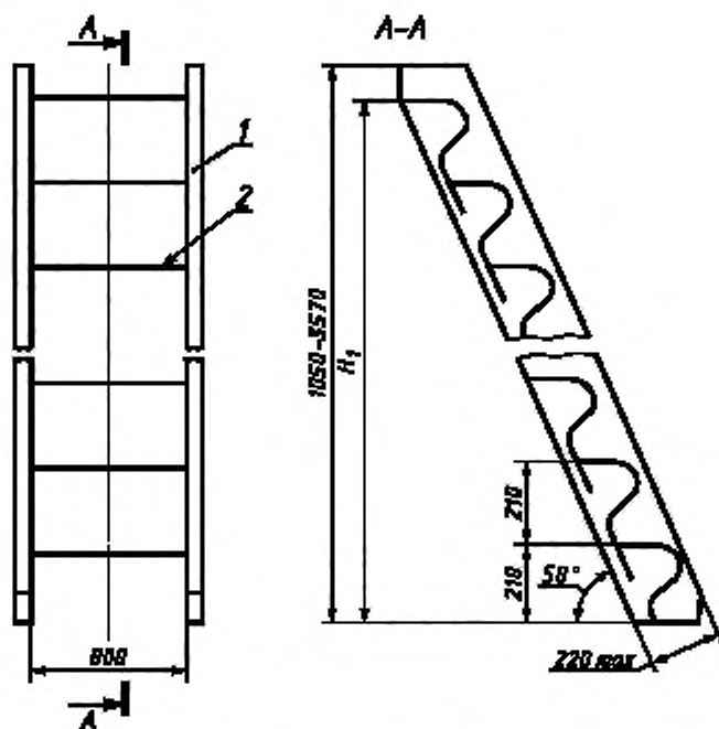
Масса 1 м стального трапа — 62,0 кг 1 — тетива; 2 — ступенька
