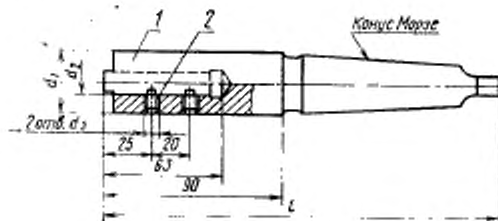
1—оправка; 2—винт по ГОСТ 1477-75
