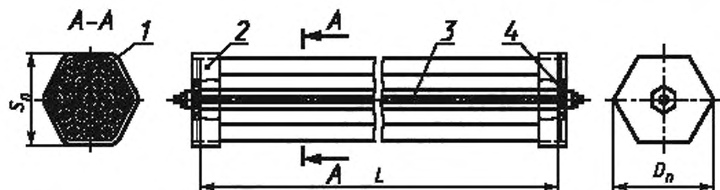
D_n — диаметр пакета, S_n — ширина пакета, L — длина трубы в пакете 1 — буровая труба; 2 — крышка; 3 — стяжка; 4 — прокладка деревянная Черт. 6
