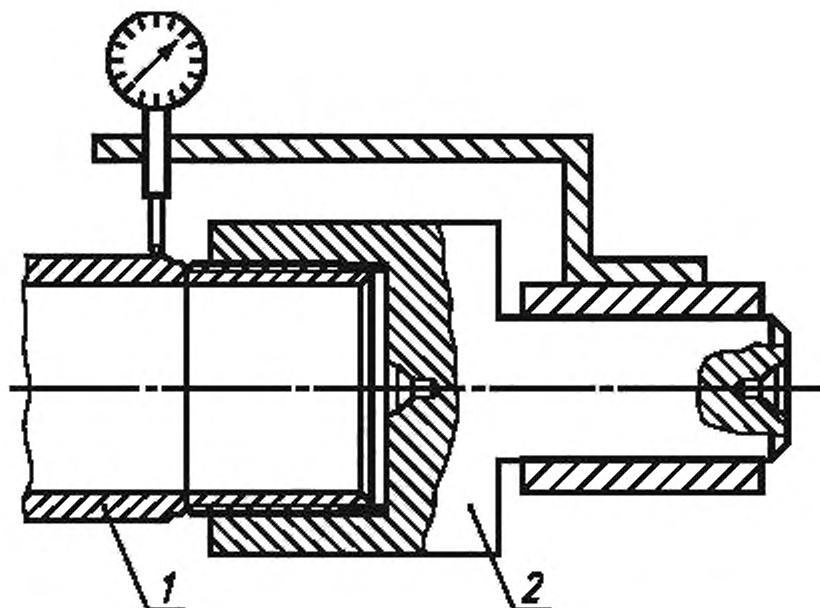
1 — труба, 2 — оправка
