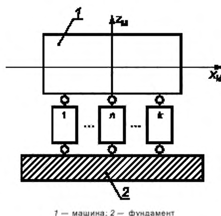
Рисунок 1 — Аналитическая модель машины, установленной на виброизоляторы
