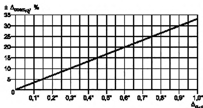
Рисунок В.1 — Зависимость максимальной погрешности \pm \Delta_{\cos \alpha_{Fq}} от угла сдвига фаз между измерительными каналами силы и скорости при \alpha_{Fq \max} = 87^\circ
