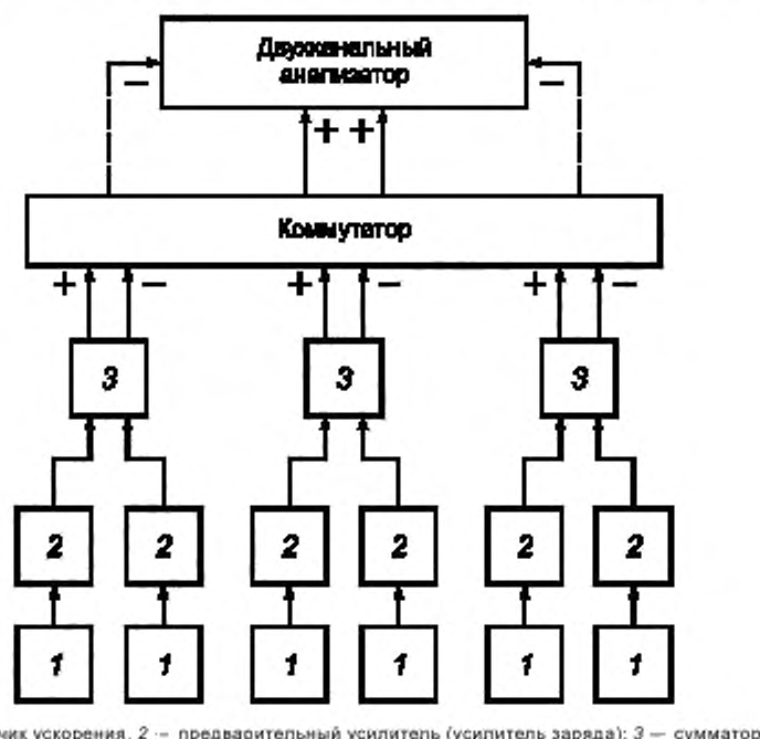
Рисунок 5 — Схема типичного измерительного тракта для определения взаимного спектра составляющих вибрации машины и фундамента с помощью датчиков ускорения вибрации
