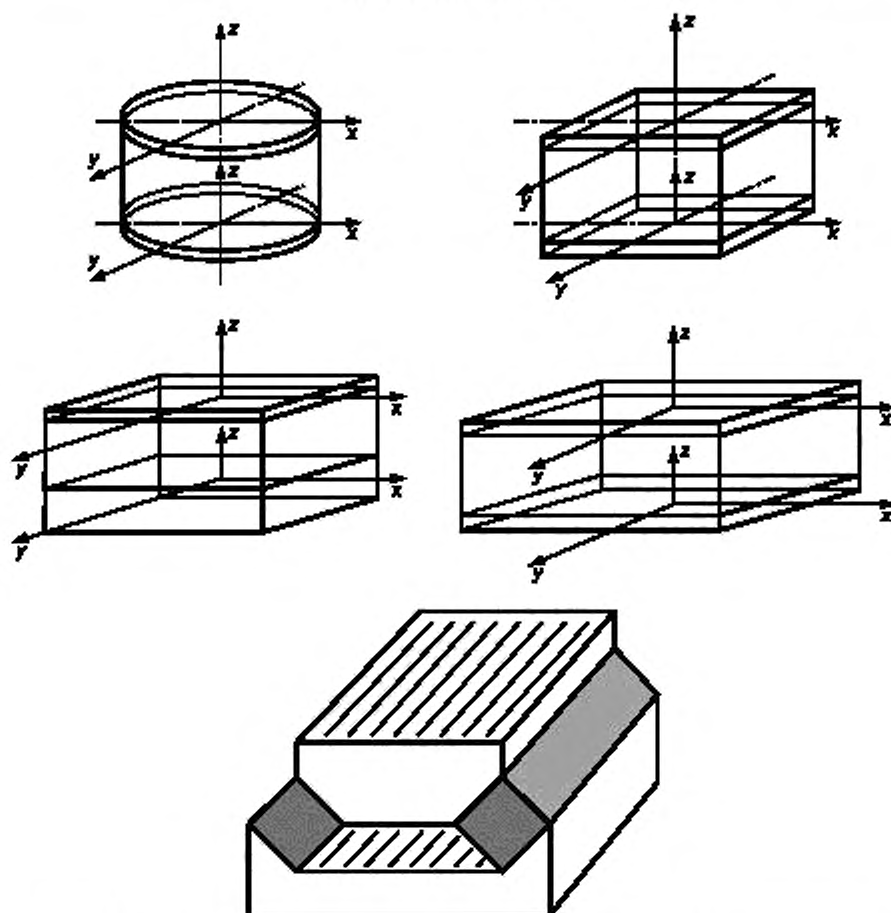
Рисунок Б.1 — Обобщенная схема осесимметричных виброизоляторов и виброизоляторов, симметричных относительно плоскостей zx и zy
