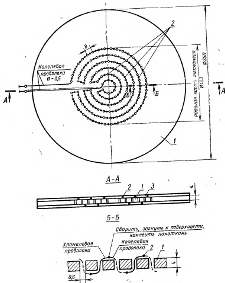
Схема тепломера
