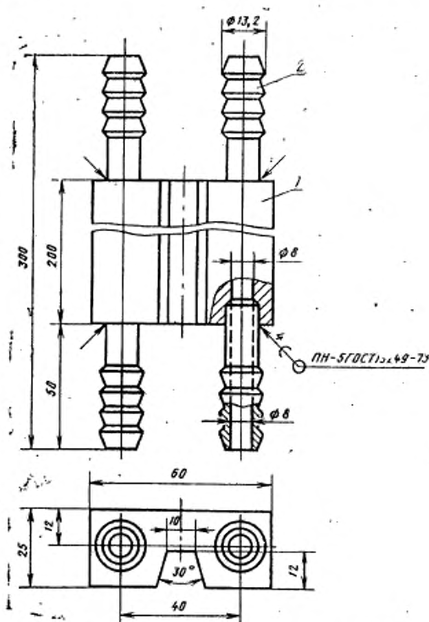
1 — корпус кристаллизатора; 2 — штангенциркуль
