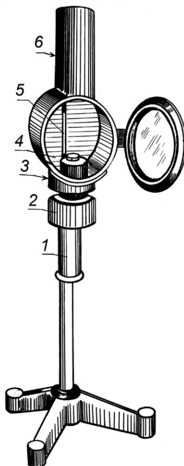
Рисунок 1 — Лампа для определения высоты некоптящего пламени
