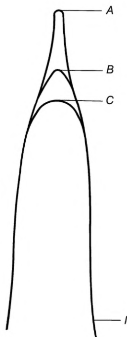
Рисунок 4 — Вид пламени
