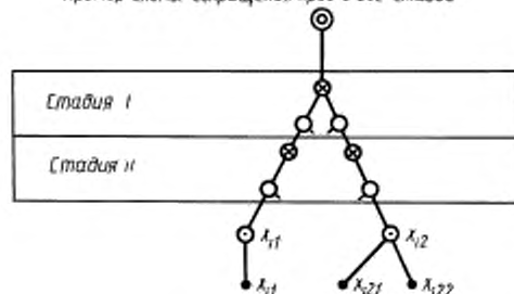
Пример схемы сокращения проб в две стадии
