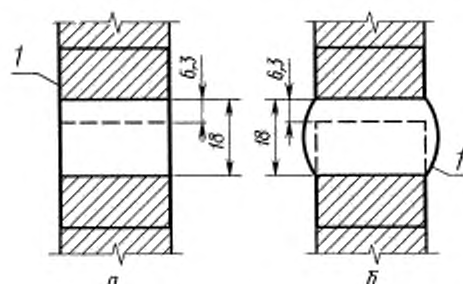
Установка увеличенного образца размером 105 \times 65 см
