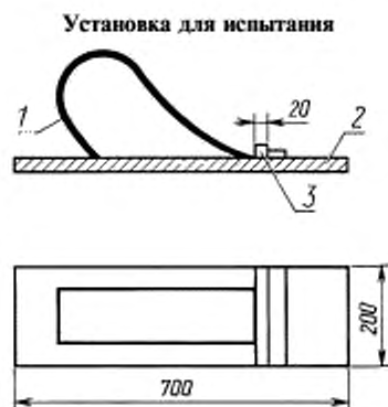
1 — образец для испытания; 2 — заплечик; 3 — стальной брусок
