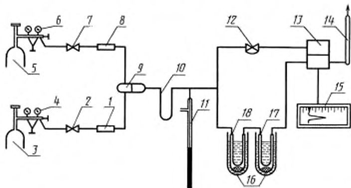
Схема установки для измерения удельной поверхности
