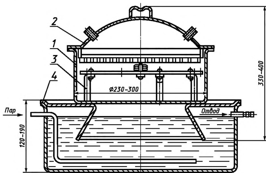
1 — корпус; 2 — крышка; 3 — подставка; 4 — водяная баня
