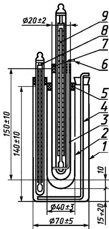
1 — стакан; 2 — впаиваемая пробирка; 3 — пробирка; 4, 6 — мешалки; 5, 7 — пробки; 8 — термометр; 9 — специальный термометр
