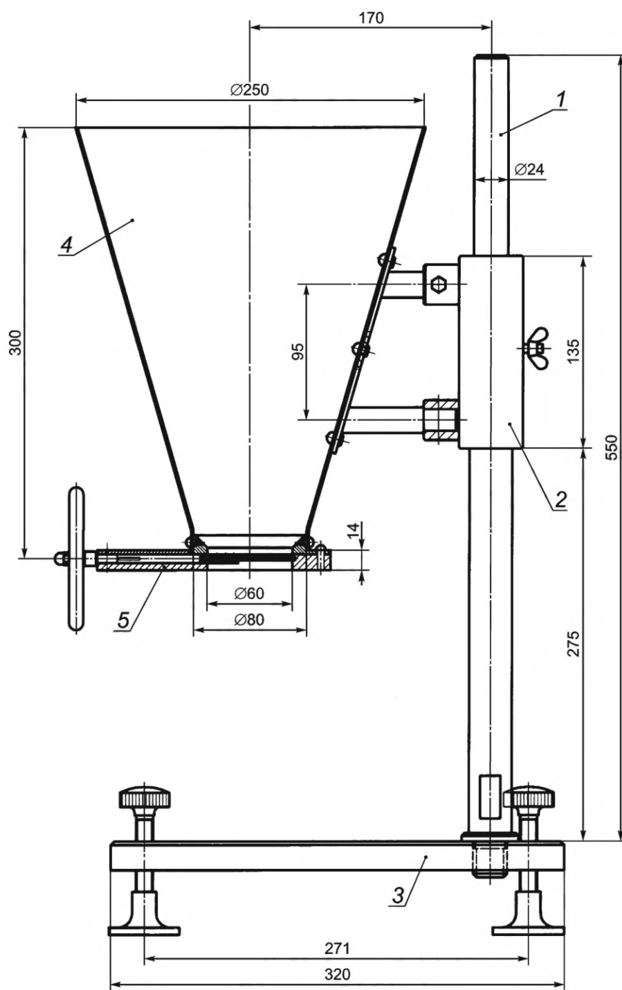
1 — стойка; 2 — втулка; 3 — плита; 4 — бункер; 5 — шибер с заслонкой
