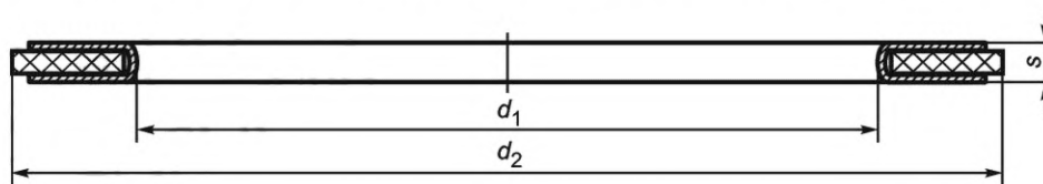
Рисунок 2 — Неметаллическая прокладка с фторопластовым чехлом
