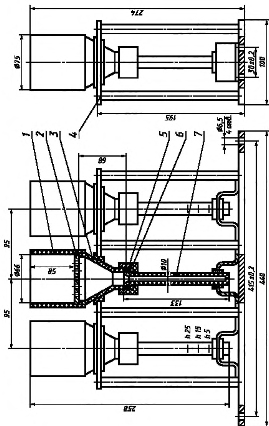
1 — камера; 2 — сито; 3 — воронка; 4 — корпус в сборе; 5 — прокладка; 6 — гайка; 7 — измерительная трубка
